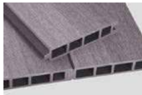
Secțiune transversală a scândurii l 28 mm
